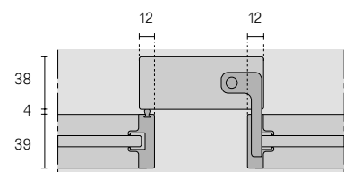
Sistema di scorrimento con trascinio Sliding system with connecting plate
